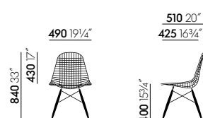
Wire Chair DKW, scocca in fili metallici, basamento in legno con montanti in acciaio tubolare
