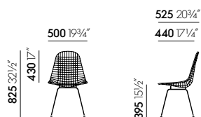
Wire Chair DKX, scocca in fili metallici, basamento tubolare d'acciaio con quattro gambe
