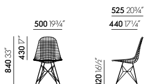
Wire Chair DKR, basamento e scocca in fili metallici
