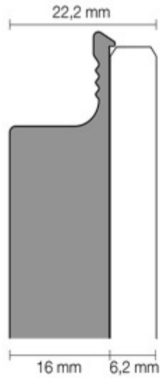
Sezione Laminam / Pietre Luxury : Section Laminam / Pierres Luxury :
