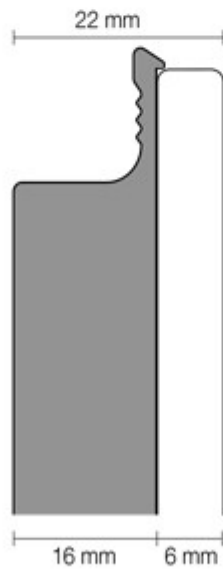
Sezione Laccato: Section laqué :
