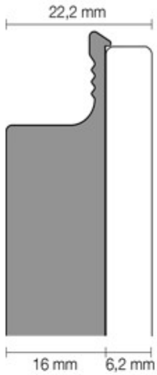
Sezione Corian: Section Corian :
