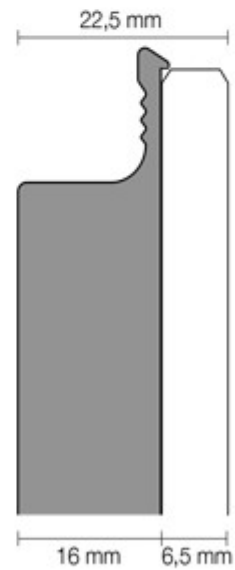
Sezione Laminato, Fenix: Section Stratifié, Fenix :
