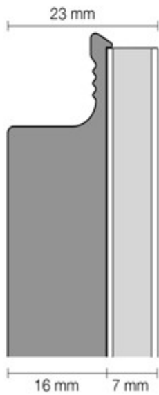
Sezione Aludust: Section Aludust :
